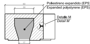
SECCIÓN B-B' / SECTION B-B'
